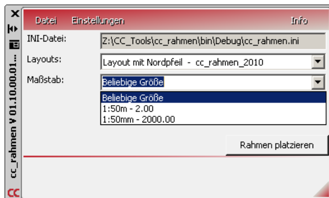
Programmdialog
