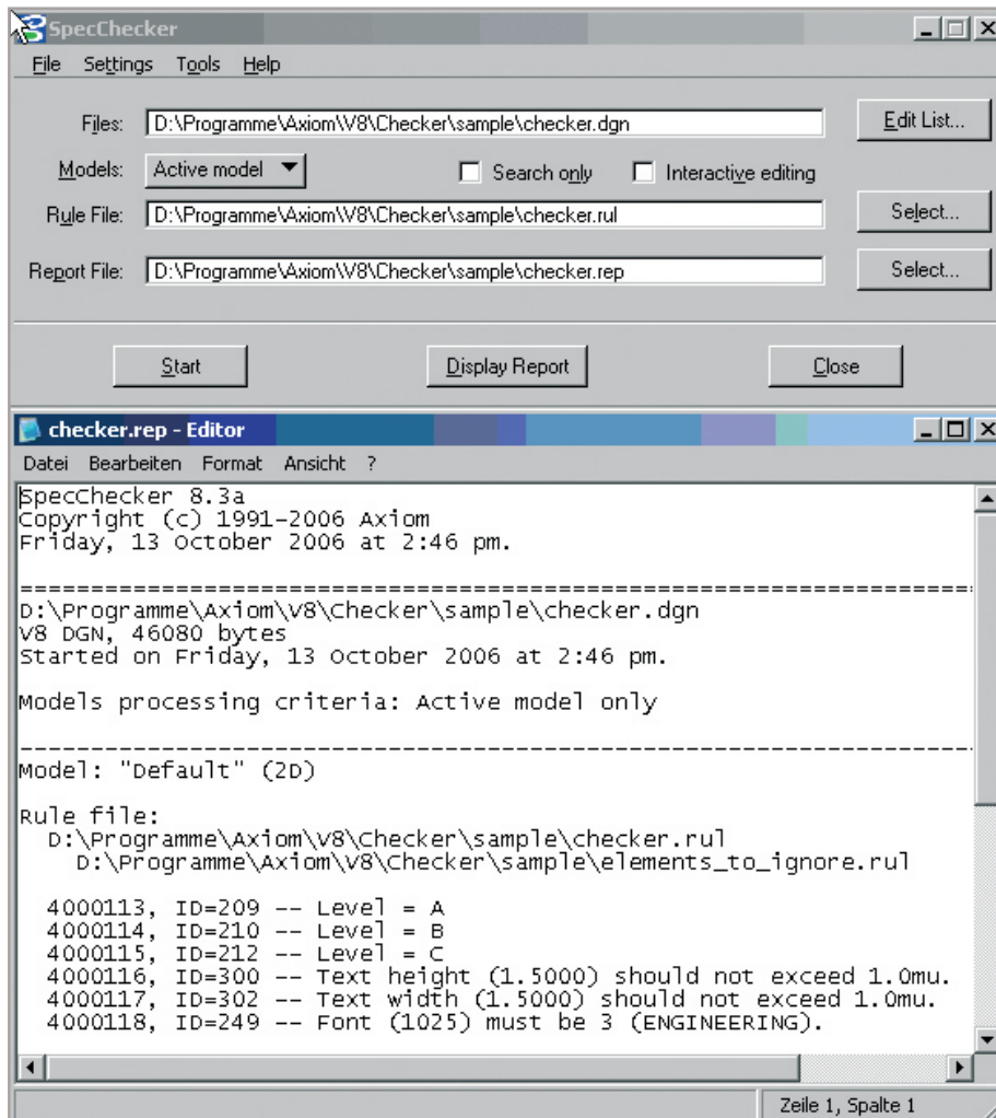
SpecChecker: Beispiel
