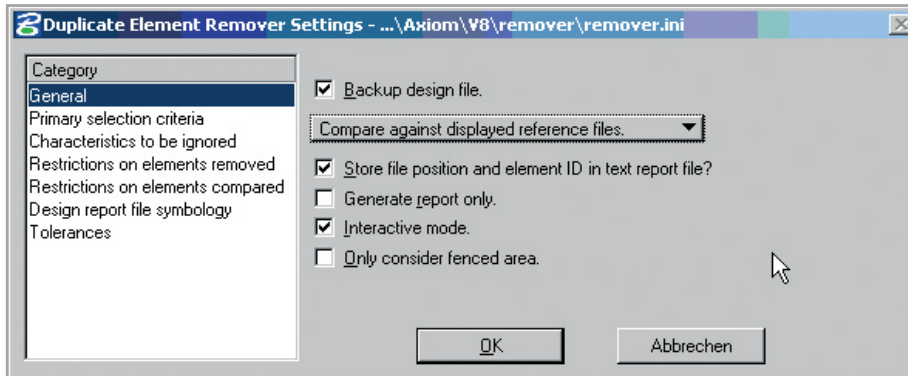
DuplicateElementRemover
